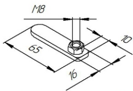
Закладной кронштейн z-47 М8_10
