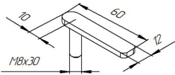
Закладной кронштейн z-32 М8х30_10
