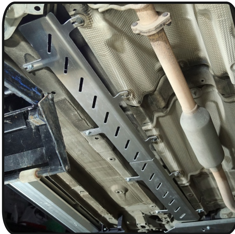
Защита топливопровода (алюминий) 4 мм (2шт) арт.ZKTCC00627.
