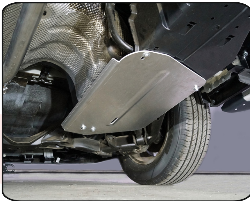
Защита бака (алюминий) 4мм арт. ZKTCC00603
