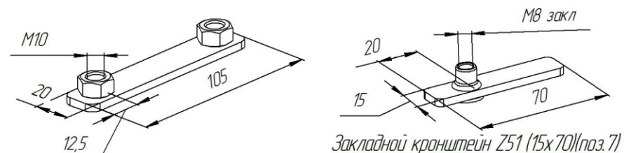
Закладной кронштейн Z68 (20x105)(поз.8)
