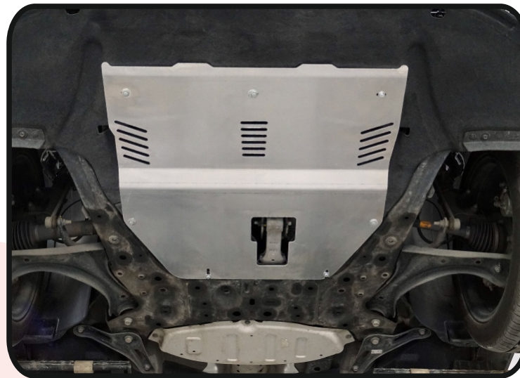
Защита картера (алюминий) арт. ZKTCC00438.
