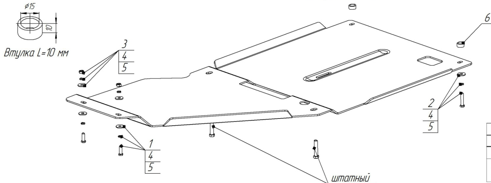
Схема установки
