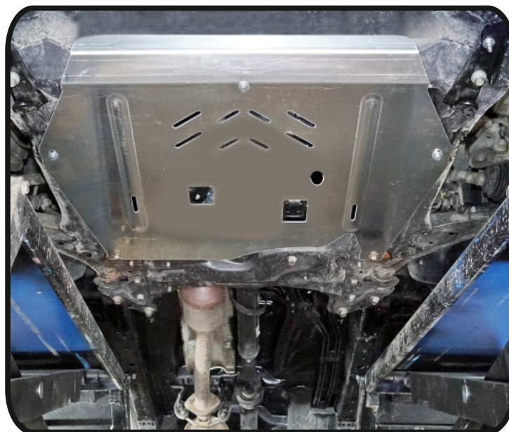
Защита картера и КПП (алюминий) 4мм арт.ZKTCC00404
