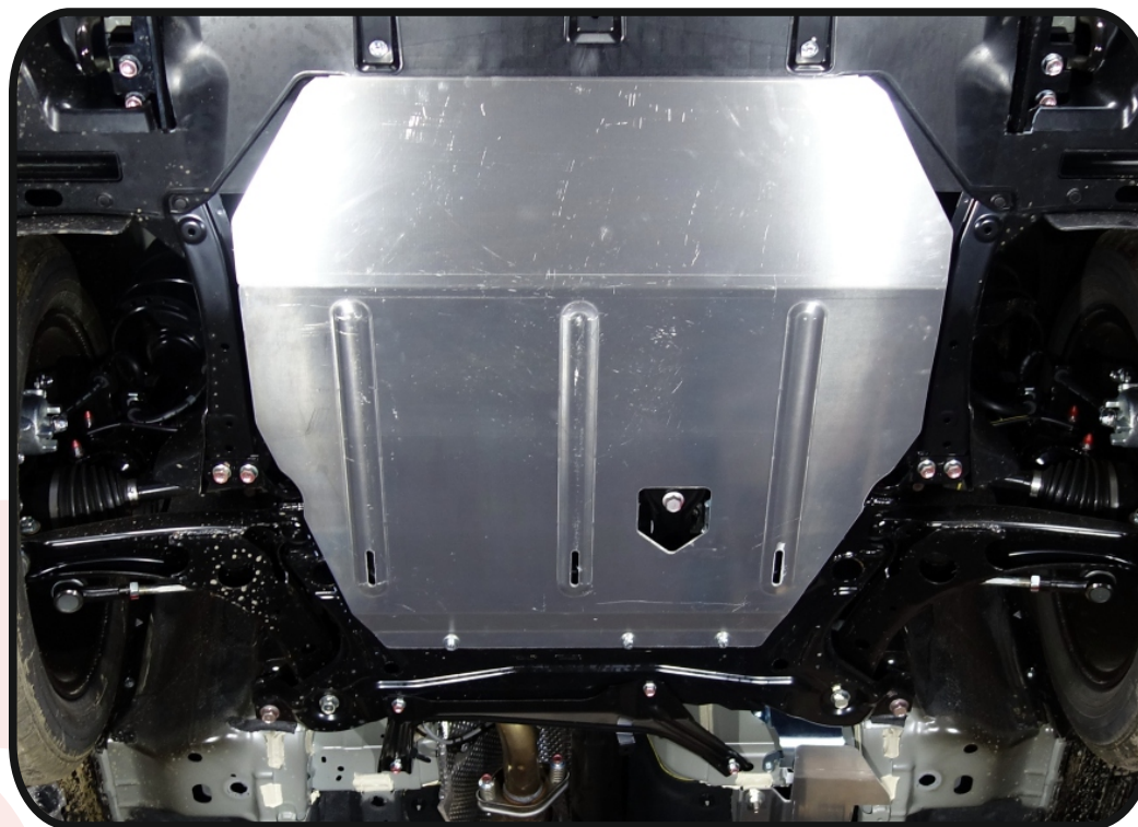
Защита картера и КПП (алюминий) 4 мм арт. ZKTCC00346
