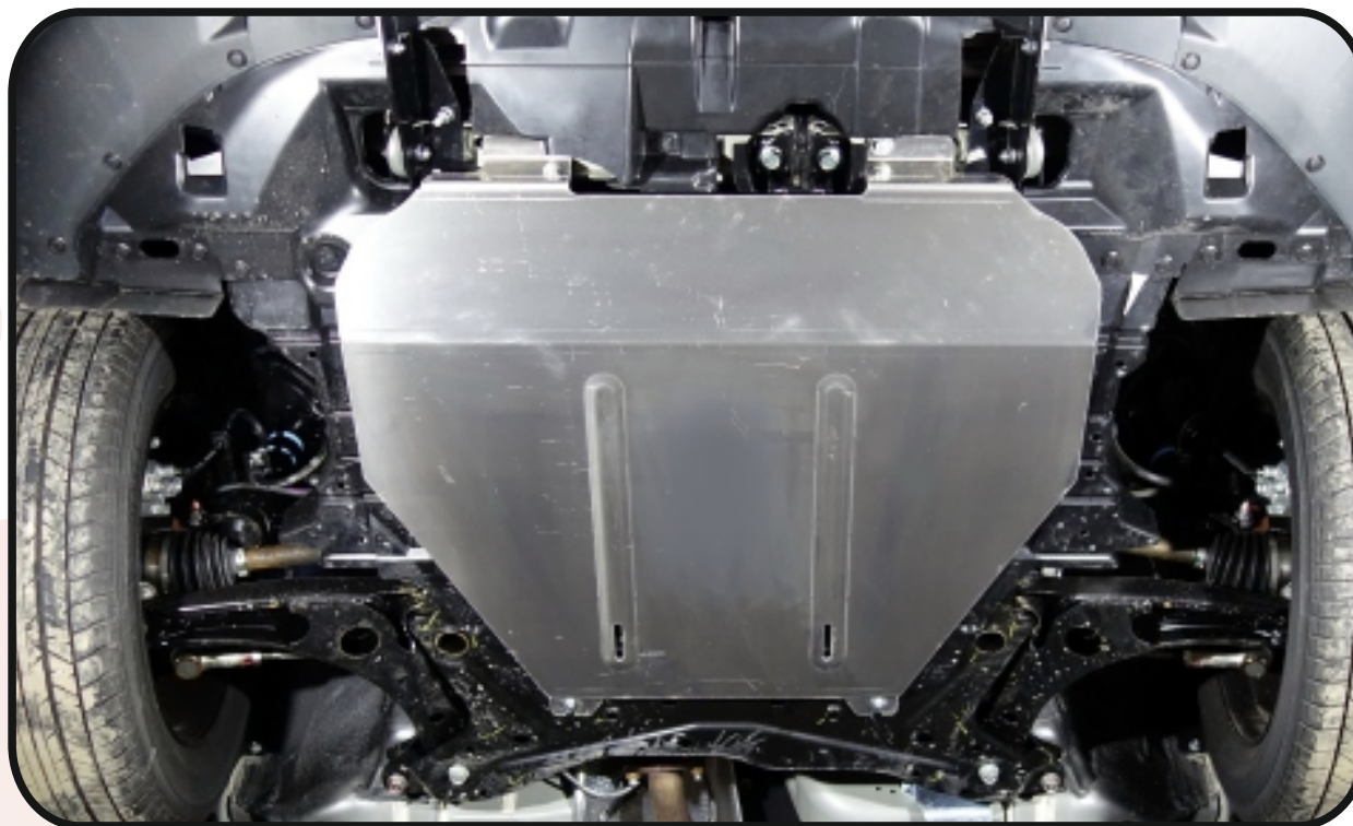
Защита картера и КПП (алюминий) 4 мм арт. ZKTCC00334.
