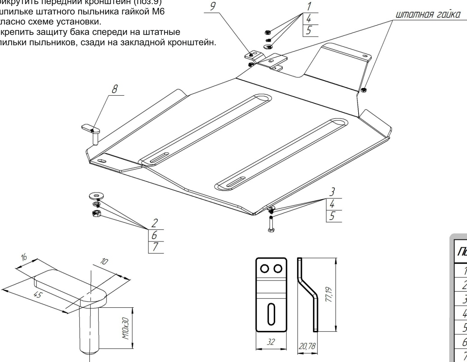
Закладной кронштейн М10х30 (поз.8)
