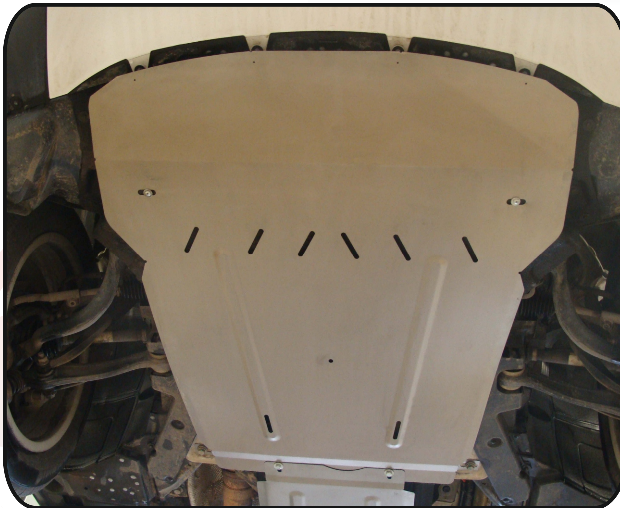
Защита картера (алюминий) 4 мм арт. ZKTCC00192.
