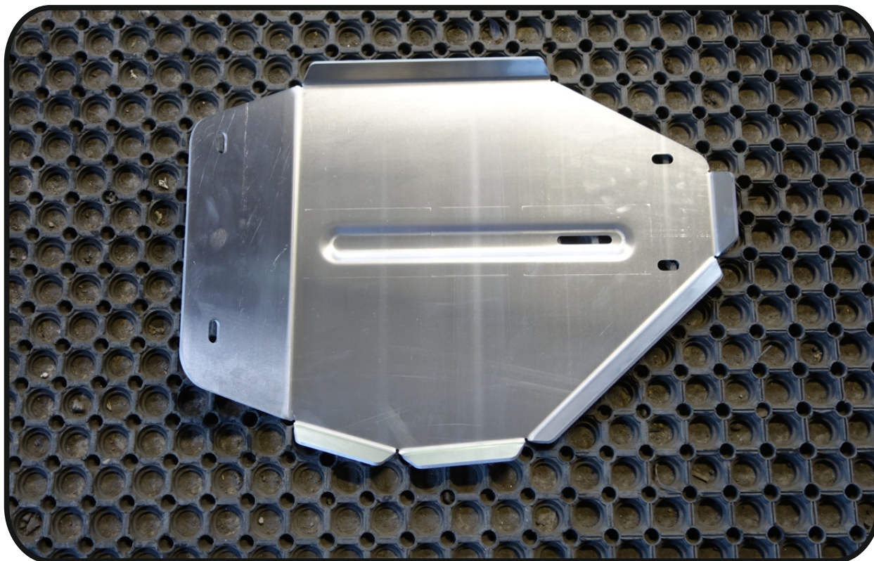
Защита бака (алюминий) 4мм арт.ZKTCC00172
