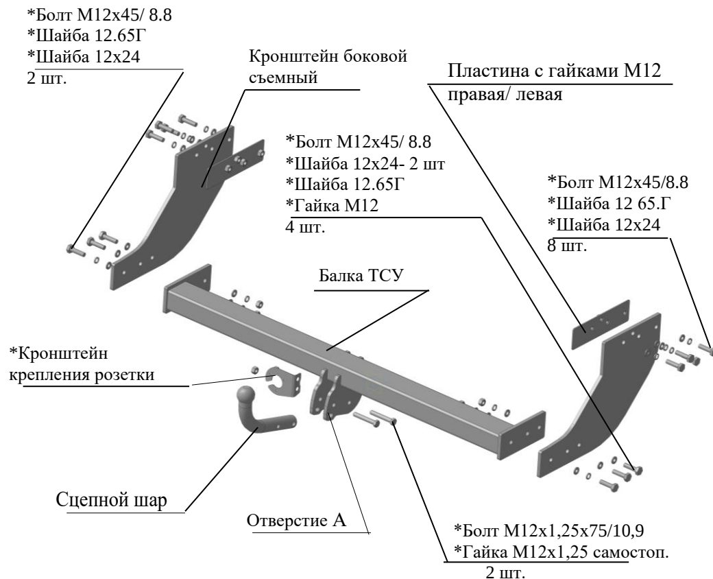
Рис.1 Тягово-сцепное устройство ТСУ 8124.
