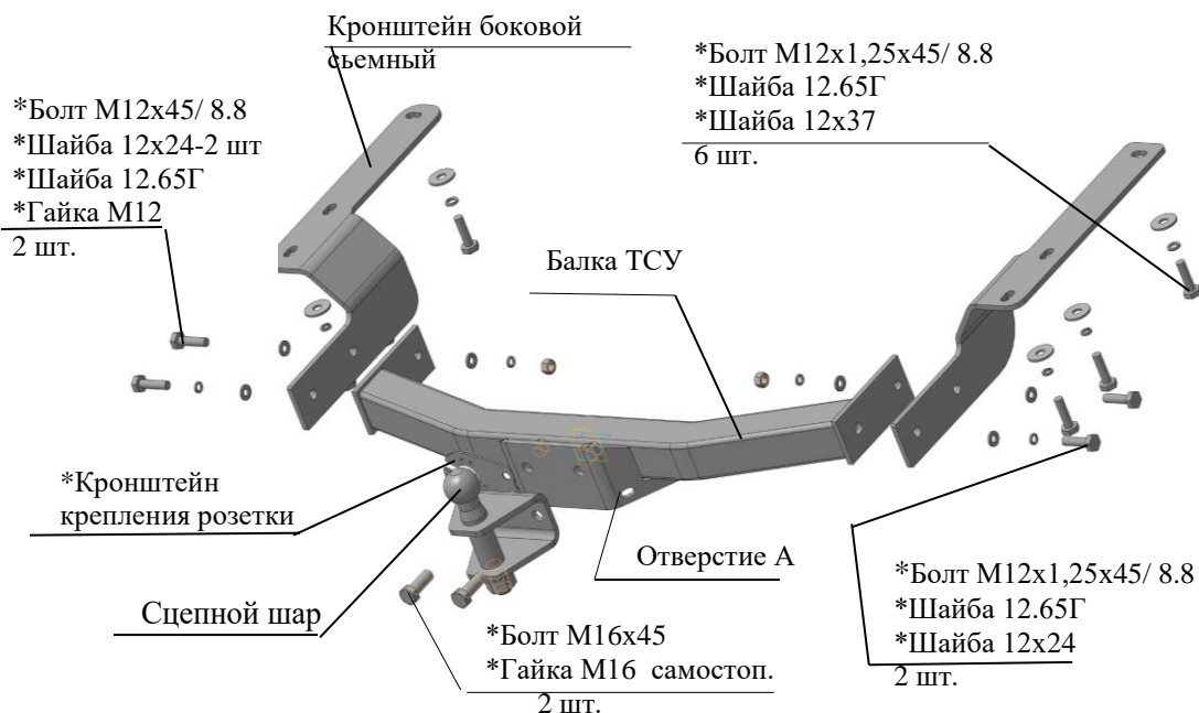
Рис.1 Тягово-сцепное устройство ТСУ 7850.
